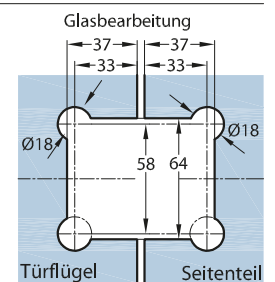
Türflügel
